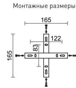
Монтажные размеры
