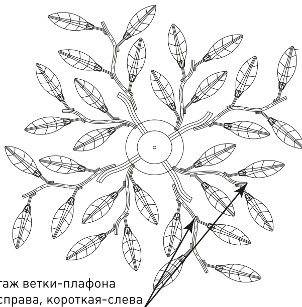
Вид сбоку собранной люстры
