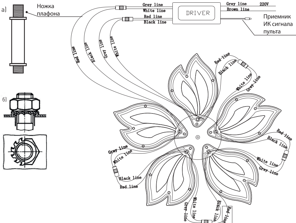
(Рис.2). На схеме соединения проводов указан цвет проводов соединения.
