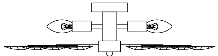
Вид сбоку собранной люстры
