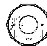
Отверстия для монтажа ALMAZ RGB 25W R
