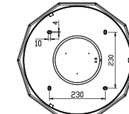
Отверстия для монтажа ALMAZ RGB 60W R
