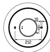
Отверстия для монтажа SATURN RGB 25W R
